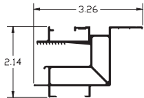
2" Retro Frame ITEM NO. SC2138
